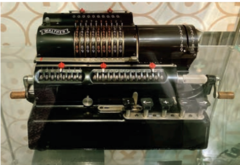
Rechenmaschine (Foto: I. Kügler)
